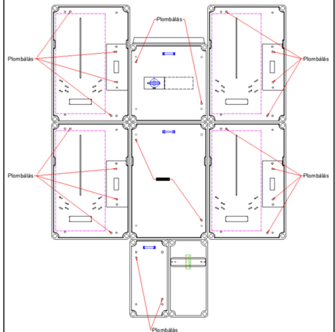
ELRENDEZÉSI RAJZ PLOMBÁLÁSI HELYEKKEL (kizárólag jó minőségű):
